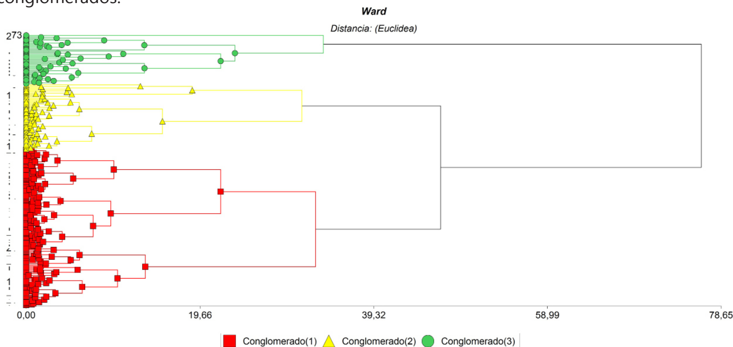
Figura 3. Dendrograma del análisis de conglomerados, según la técnica de Ward, para 224 fincas de la zona centro del Tolima.
