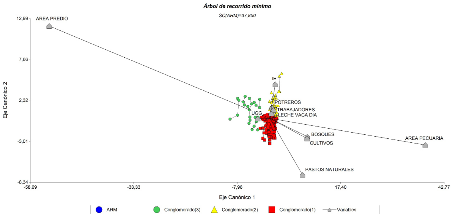
Figura 4. Árbol de recorrido mínimo.
