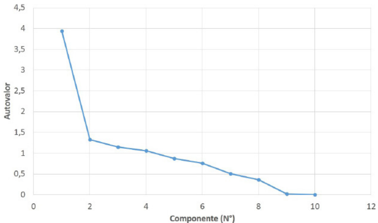
Figura 1. Método de extracción de análisis de componentes principales, rotación Varimax con normalización Kaiser.
